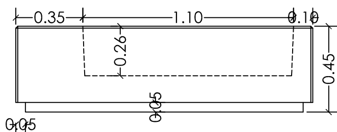
ALZADO FRONTAL Y POSTERIOR
