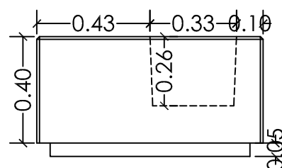
ALZADO LATERAL
