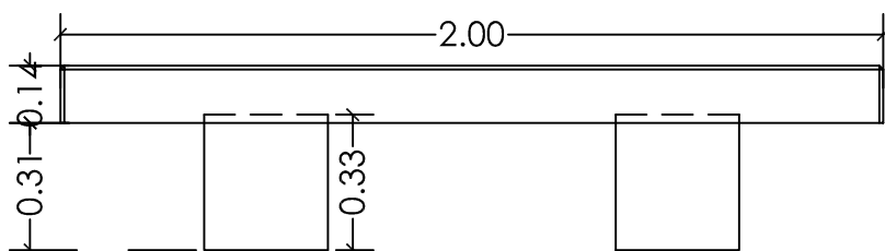
ALZADO FRONTAL Y POSTERIOR
