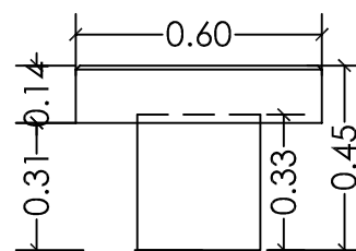
ALZADO LATERAL
