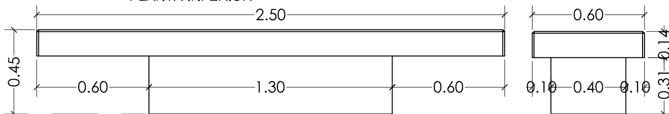
ALZADO FRONTAL Y POSTERIOR
