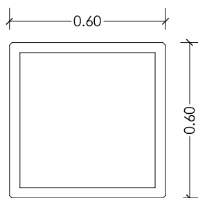
PLANTA INFERIOR
