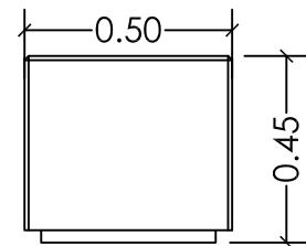
ALZADO FRONTAL
