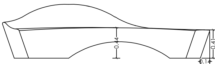
ALZADO FRONTAL
