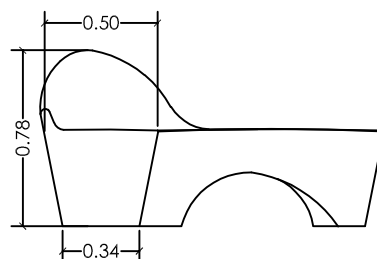
ALZADO LATERAL
