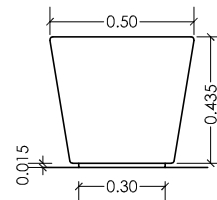
ALZADO LATERAL
