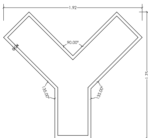
PLANTA INFERIOR
