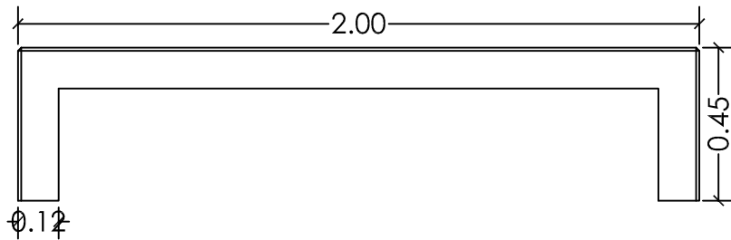
ALZADO FRONTAL
