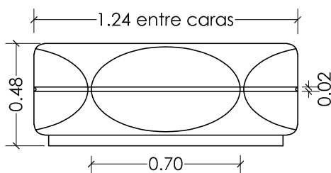
ALZADO
