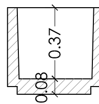
SECCION A
