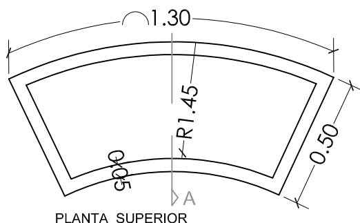
PLANTA SUPERIOR
