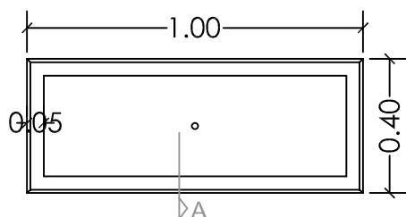
PLANTA SUPERIOR
