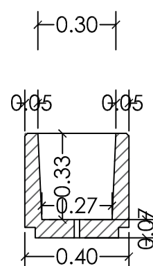
SECCION A
