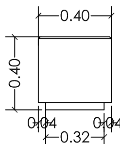
ALZADO LATERAL
