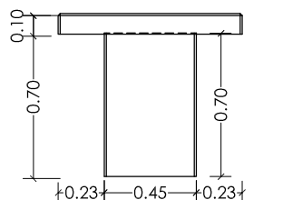
MESA ALZADO TRANSVERSAL
