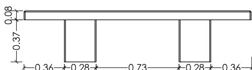
BANCO ALZADO LONGITUDINAL
