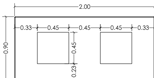
MESA VISTA INFERIOR
